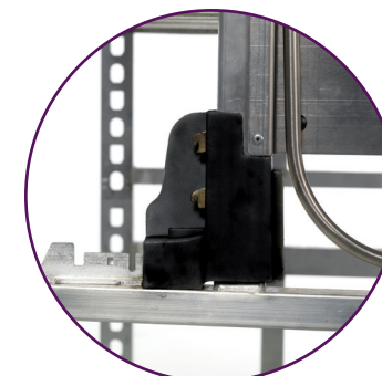
Zwarte slotplaathouder.
