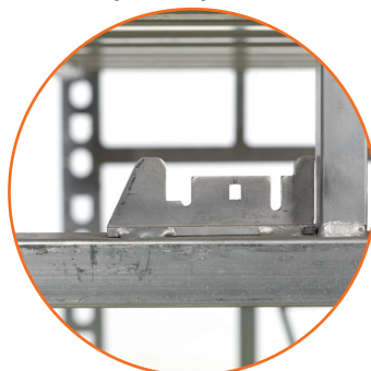
Aluminium slotplaathouder.
